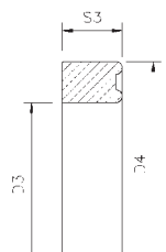
Tenuta stelo Rod seal
